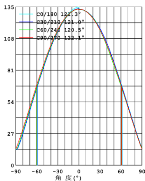
光强分布曲线
