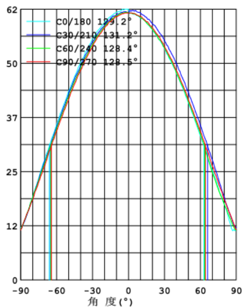
光强分布曲线
